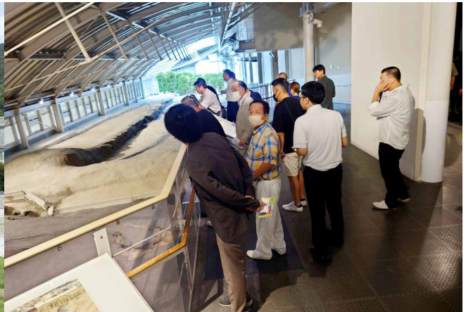
野島断層
